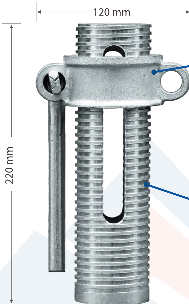
Tuerca alemana para puntal
